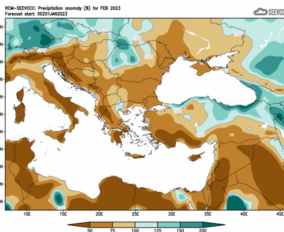
Ποσοστό μέσης μηνιαίας βροχόπτωσης (%) σε σχέση με την κανονική για τον μήνα Φεβρουάριο
