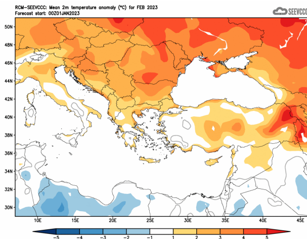
Απόκλιση μέσης μηνιαίας θερμοκρασίας (°C) από την κανονική για τον μήνα Φεβρουάριο
